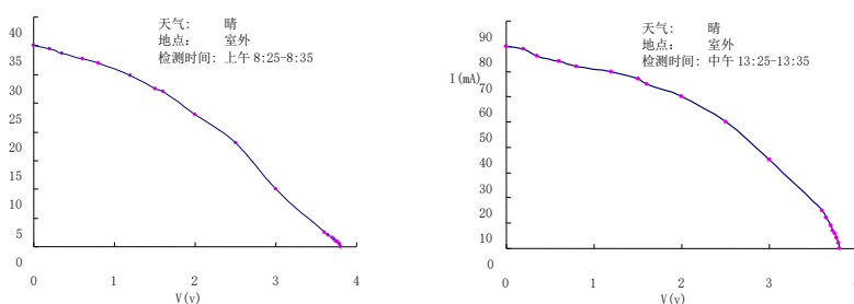
图3 小型太阳能屋顶瓦(非晶硅)晴天条件下一天测得的 I-V 曲线
