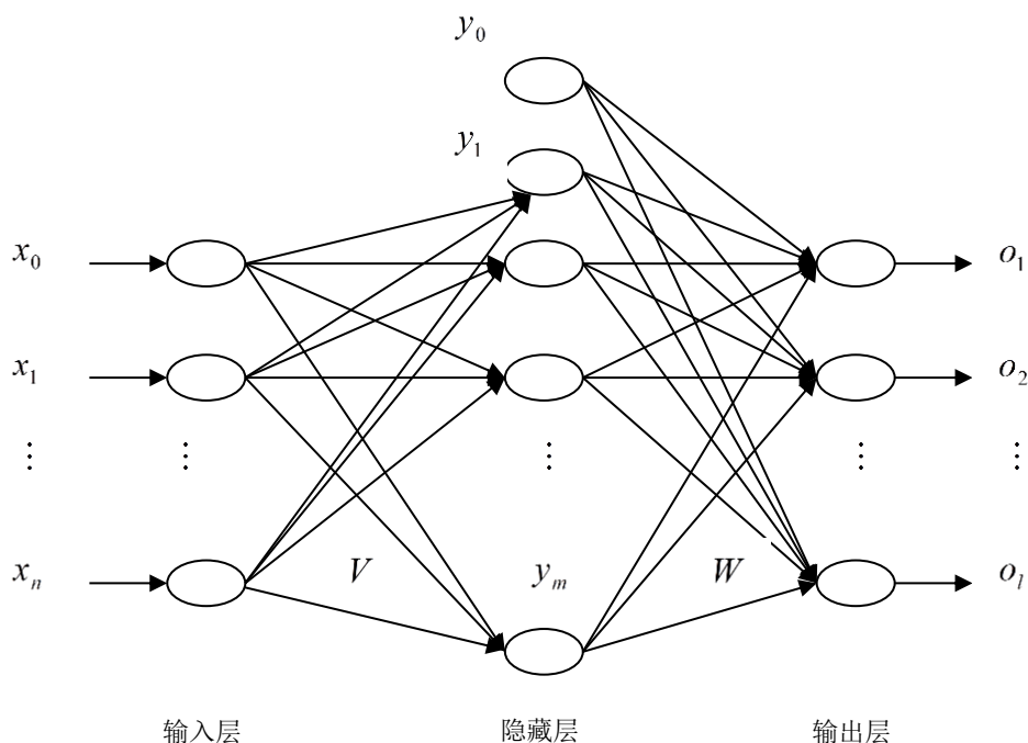
图1 BP神经网络结构
